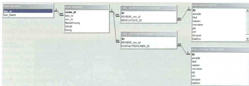
Abb. 3: Struktur der Datenbank
